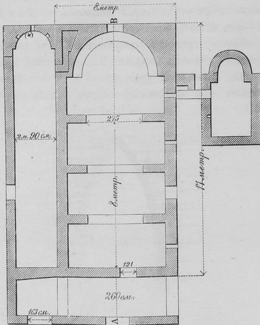
Рис. 11. Планъ церкви Тхаба-ерды.
