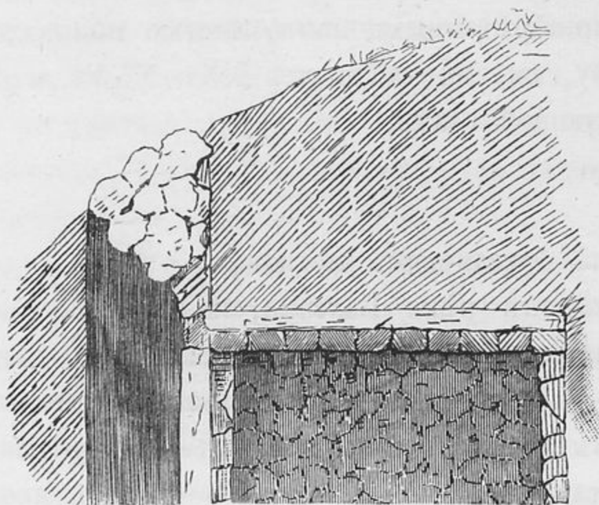
Рис. 76. Разрѣзъ склепа въ могильникѣ близъ аула Озорокова.
