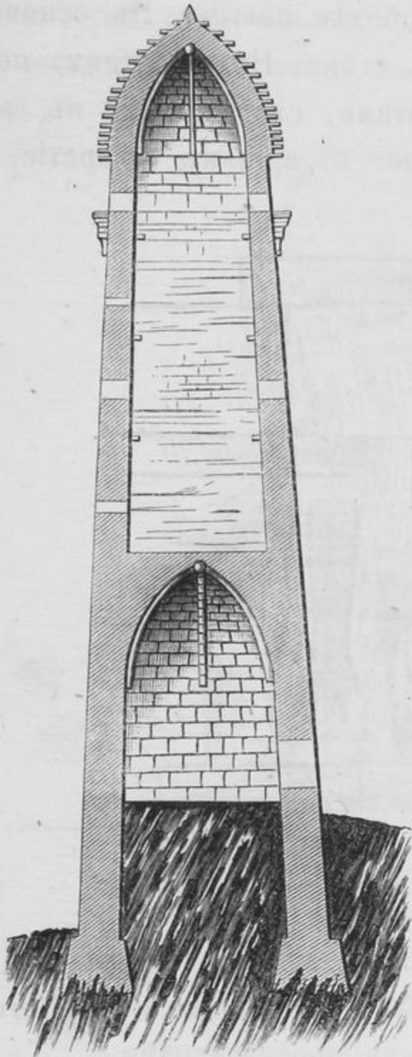
Рис. 51. Разрѣзъ башни въ Хайбахѣ.
