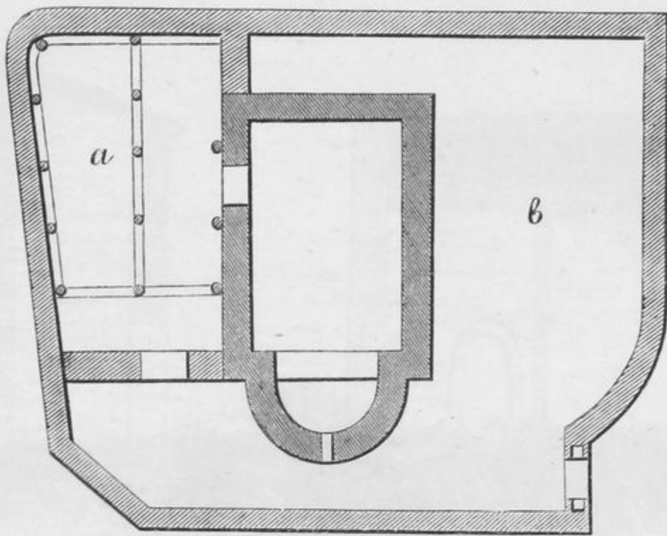
Рис. 60. Планъ дзуара въ Дзивгисѣ.
