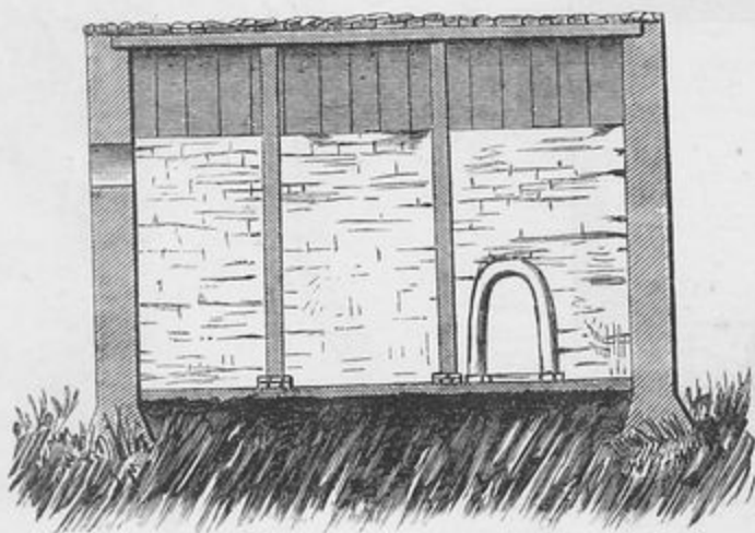
Рис. 61. Дзуаръ въ Гули въ продольномъ разрѣзѣ.
